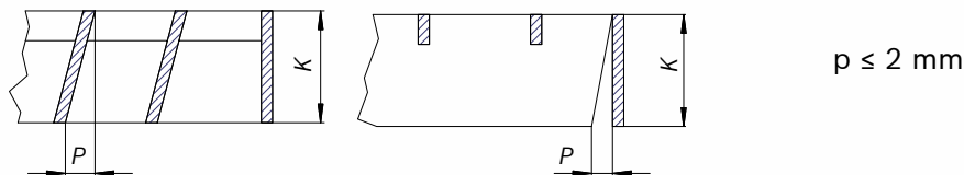
24. ábra: Főbordaferdeség, ferde végvágás
