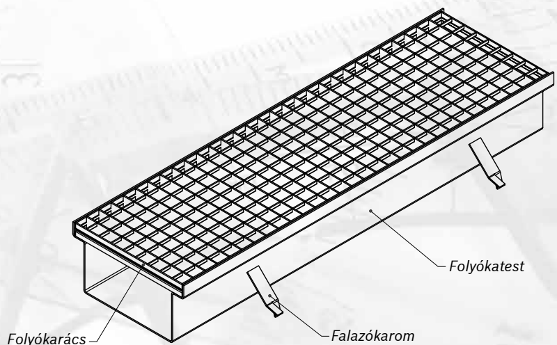
32. ábra: NC-22 típusú vízvezető
