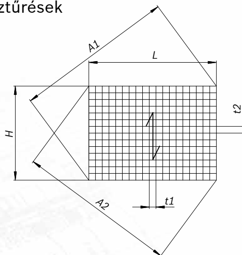
20. ábra: Normál rácsok tűrései
