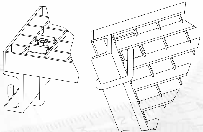
18. ábra: Horgos rögzítőszerelvény
