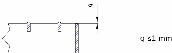
25. ábra: A mellékborða kiemelkedése
