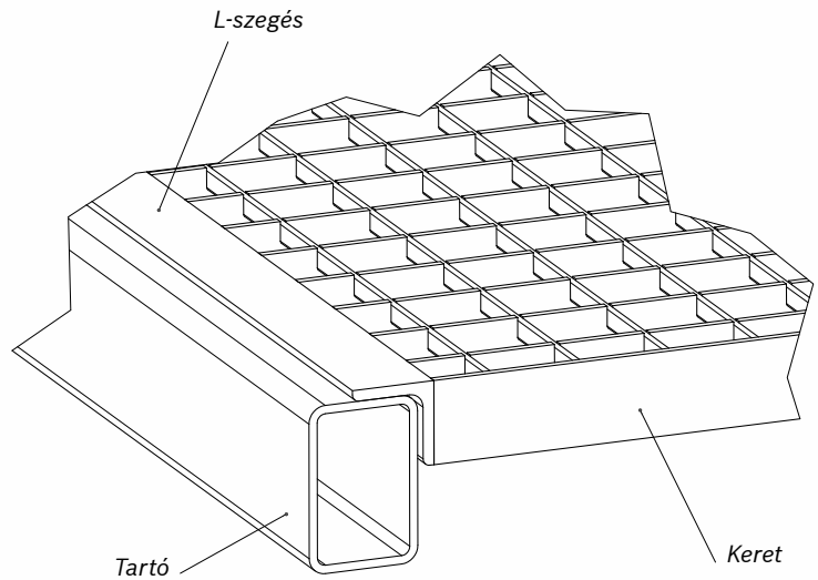
41. ábra: L-szegésű rácsok
