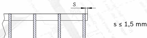
27. ábra: A mellékborða kinyúlása
