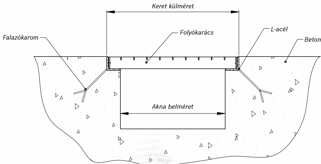
31. ábra: NC-21 típusú vízvezető
