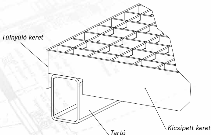
40. ábra: Polcrács kicsített kerettel
