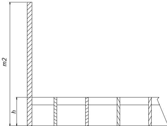
12. ábra: Bokaléc laposacélkeretes rácsra
