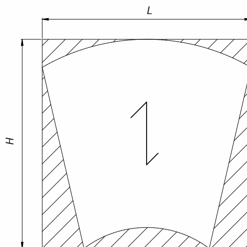
6. ábra: Alakos rácsok méretmegadása
